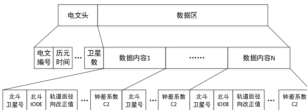
图 5-2 北斗组合轨道钟差改正电文内容编排示意图
